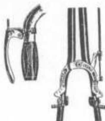
Freno Trophè posteriore da corsa chiusura laterale
